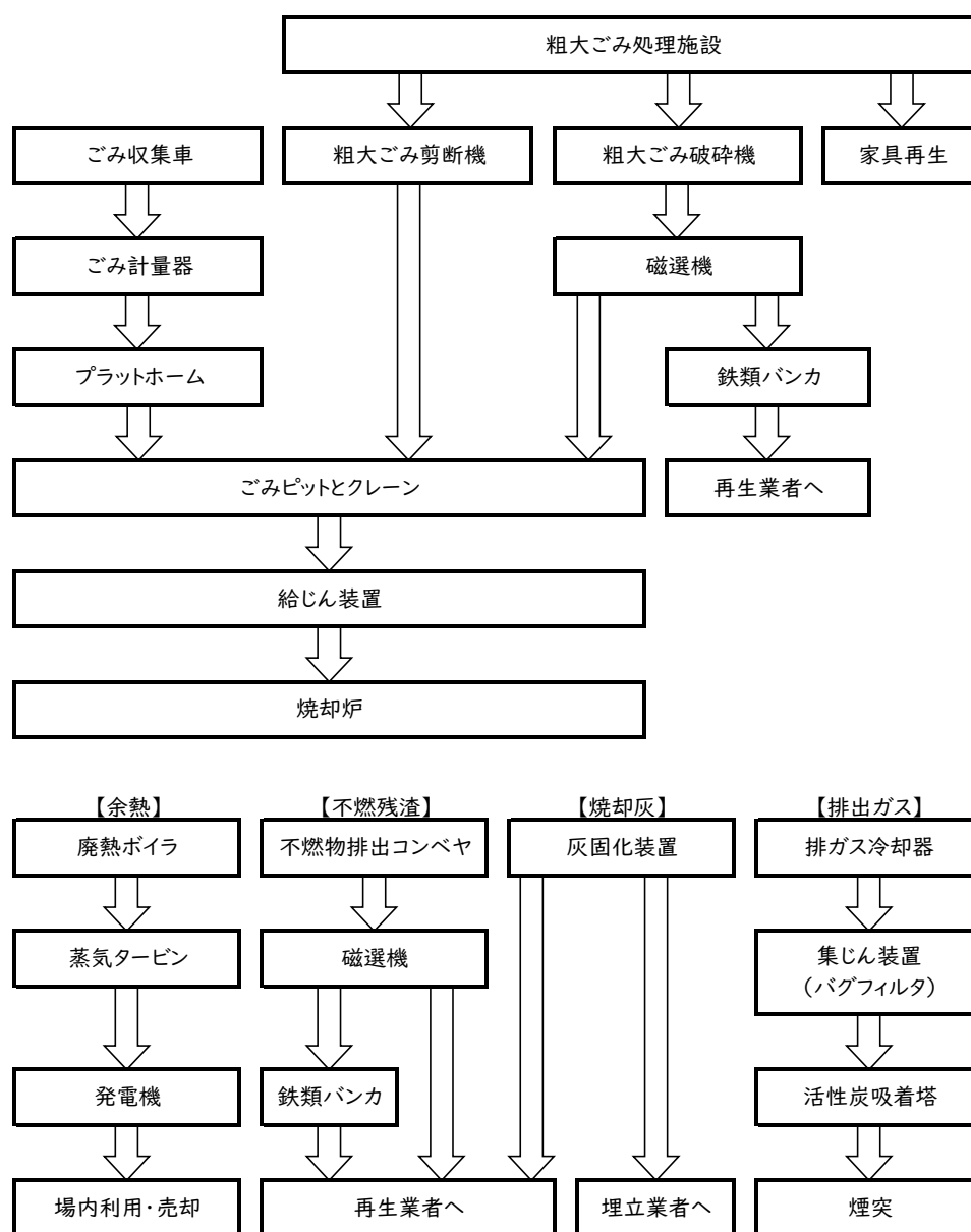
図2-3 ごみ焼却施設・粗大ごみ処理施設の処理の流れ
