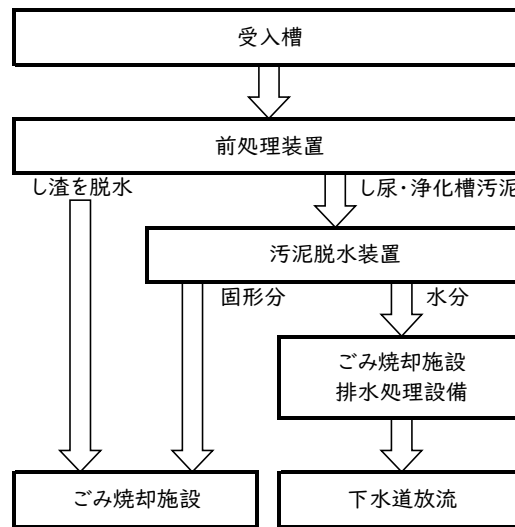
図2-10 し尿処理施設の処理の流れ
